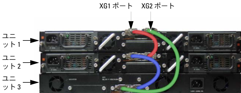
図 1-12. スイッチのスタックの接続
